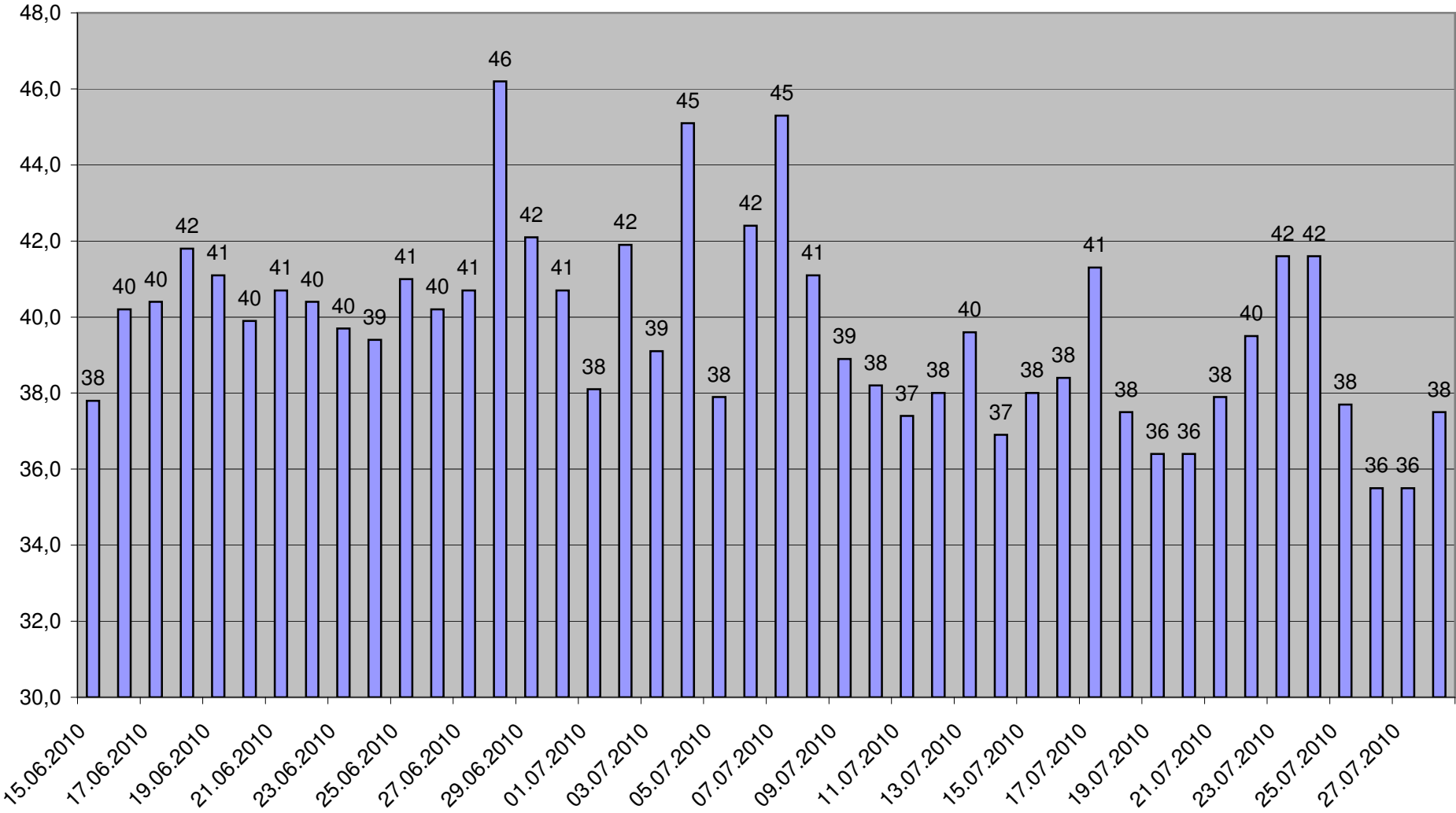
Verlauf Gesamtlärm Leq Nacht (22-6)
